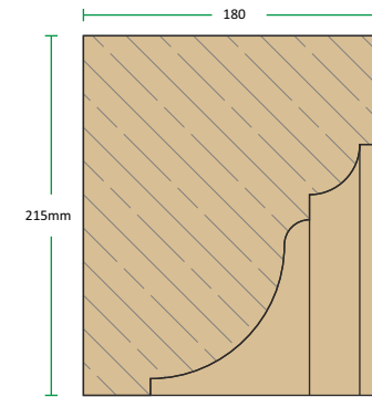
Jamb Section
